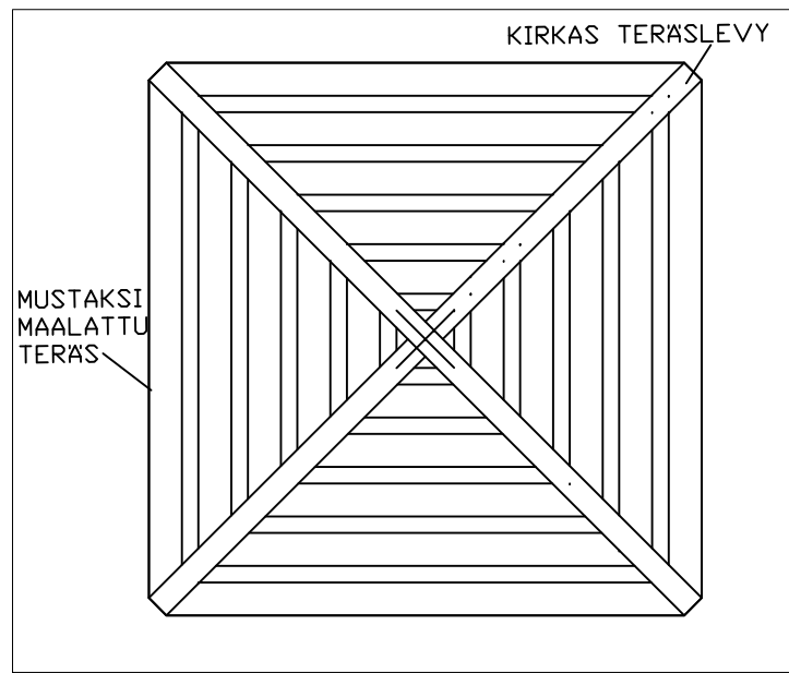
MUISTELUPAIKAN MONUMENTTI, KYNTTILÄ- JA KUKKATELINE DETALJI 1 1:50
