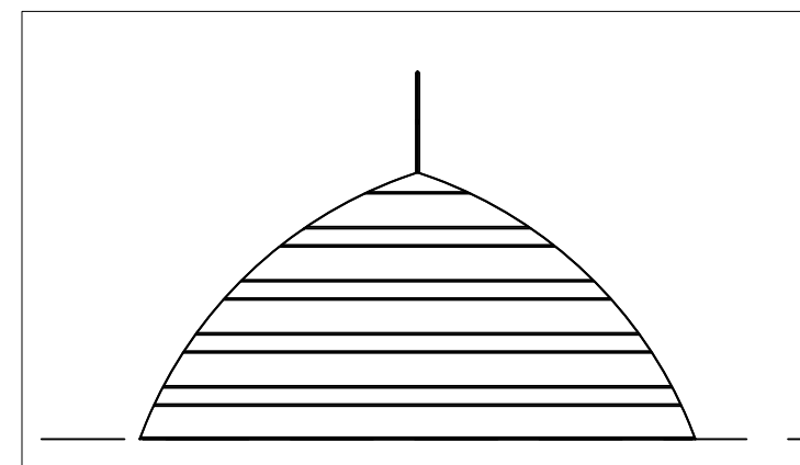
MUISTELUPAIKAN MONUMENTTI, KYNTTILÄ- JA KUKKATELINE POIKKILEIKKAUS 1:50
