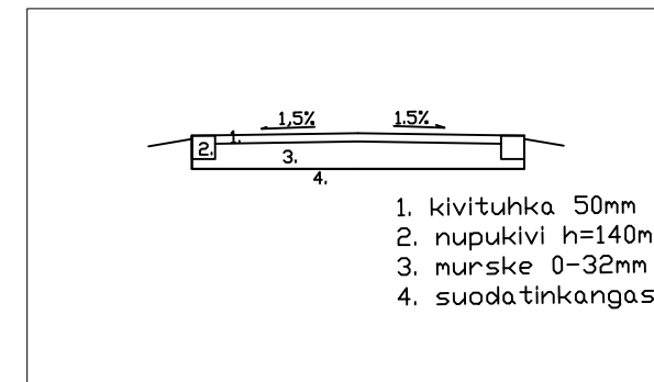
MUISTELUPAIKALLE VIEVÄN KÄYTÄVÄN POHJALEIKKAUS 1:50
