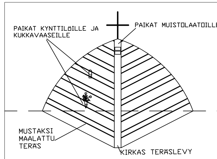
MUISTELUPAIKAN MONUMENTTI, KYNTTILÄ- JA KUKKATELINE DETALJI 3 1:50
