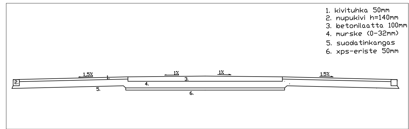
MUISTELUPAIKAN JA MONUMENTIN POHJALEIKKAUS 1:50
